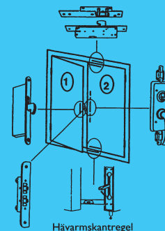
Hävarmskantregel
